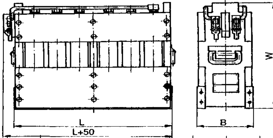
Akumulator typu KPL w obudowie z tworzywa
