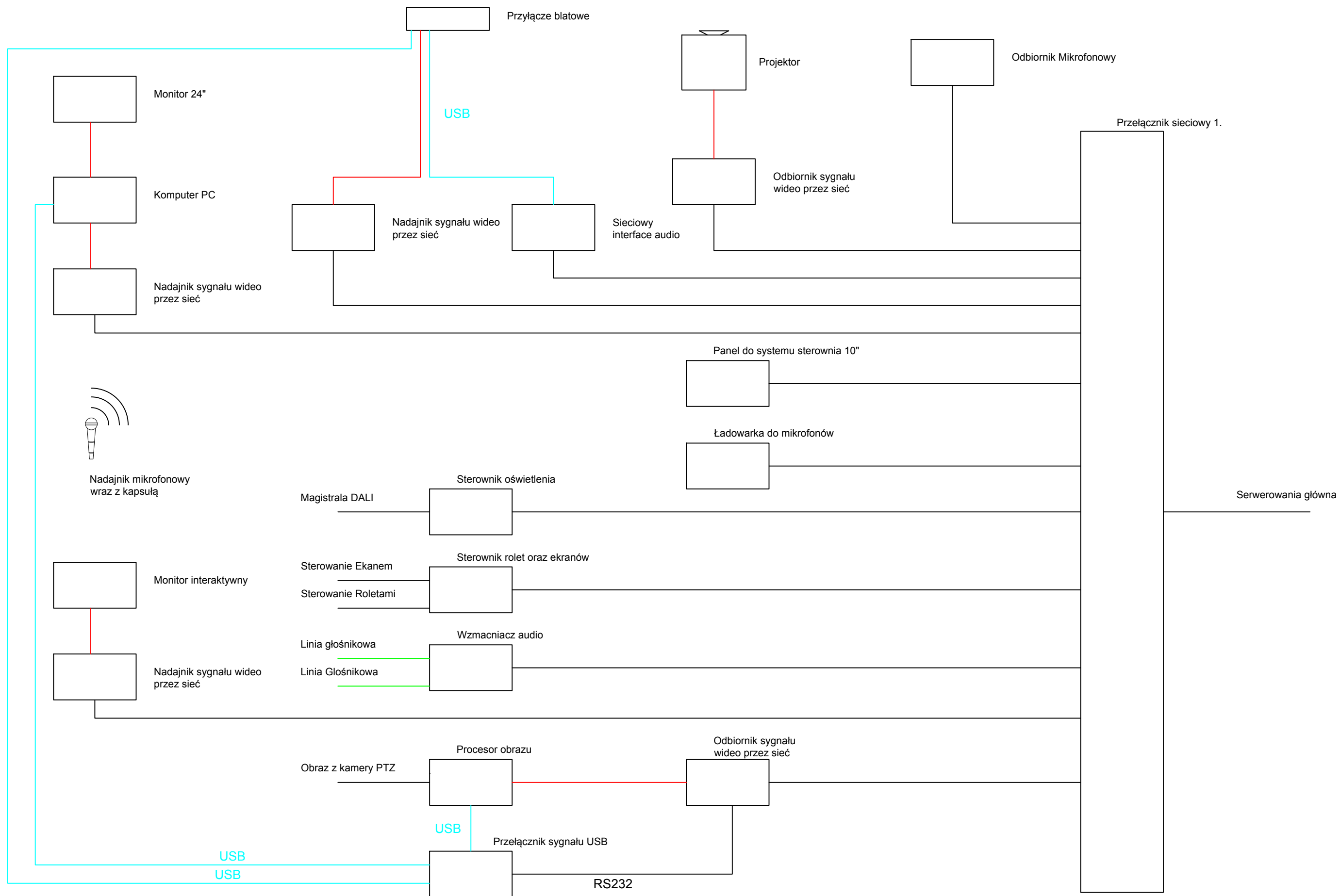
Schemat okablowania systemu AV Aula wykładowa z systemem nauczania hybrydowego
