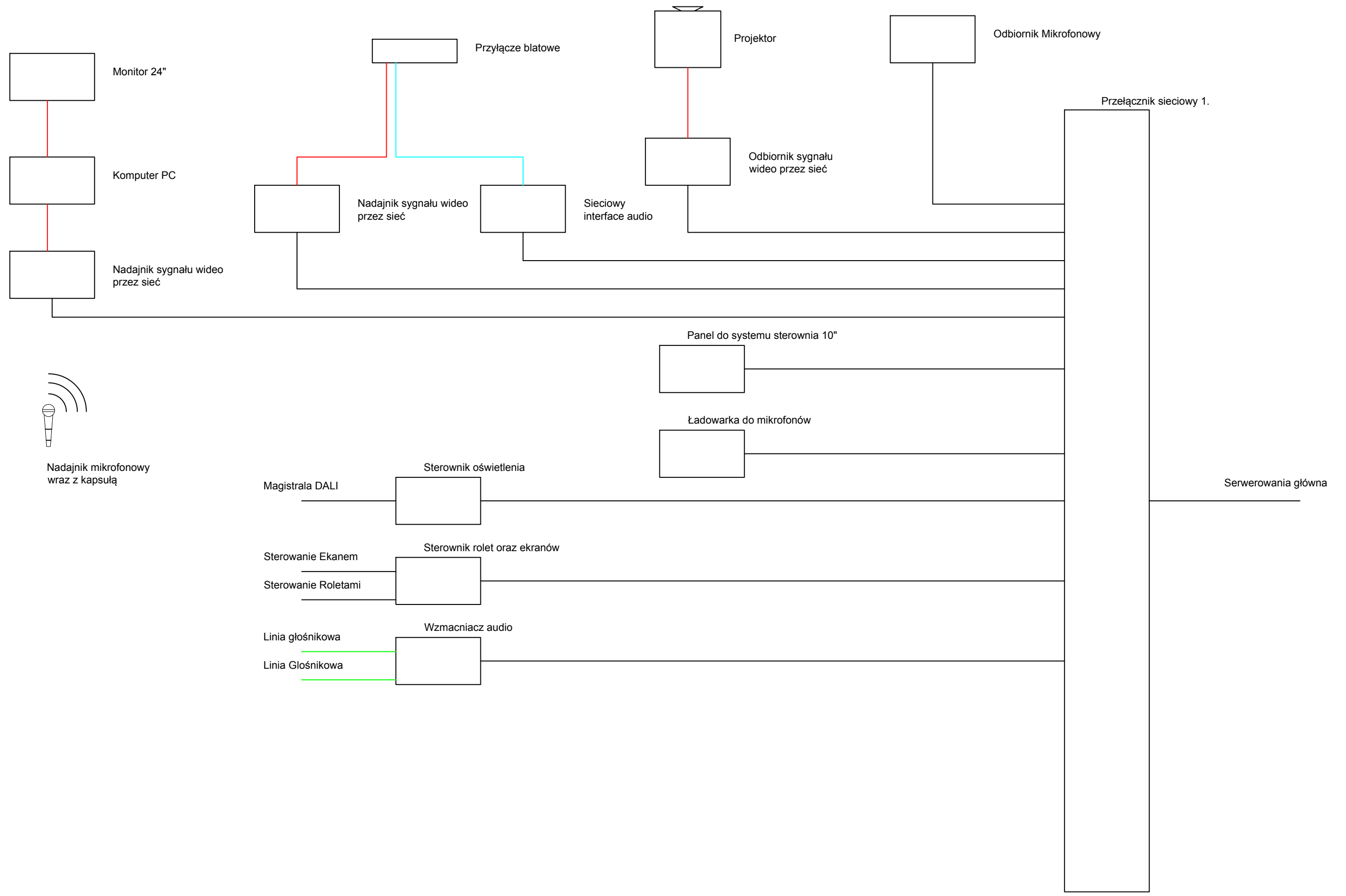
Schemat okablowania systemu AV Aula wykładowa
