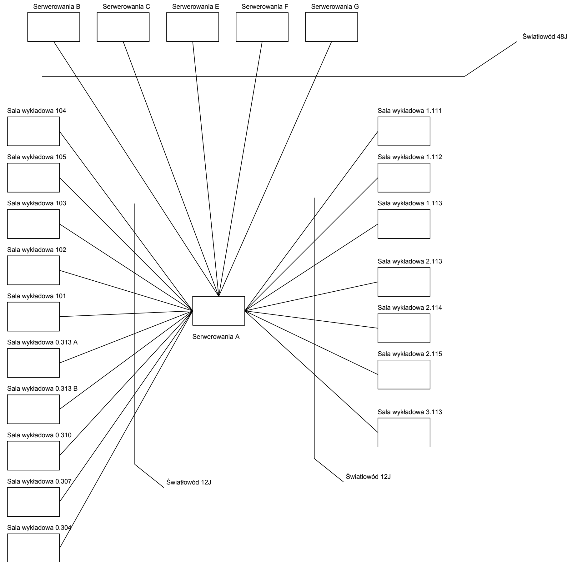
Schemat okablowania strukturalnego systemu AV
