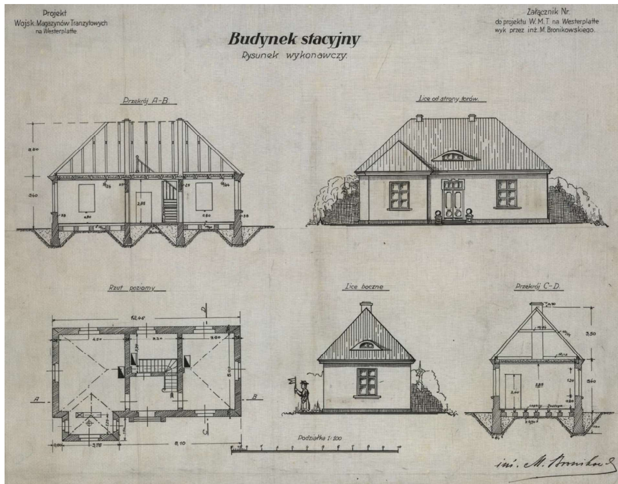
Archiwalny rysunek wykonawczy budynku zawiadowcy stacji.
