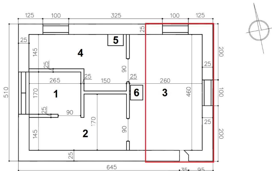
Rzut górnej kondygnacji wartowni nr 5 z przypuszczalnym rozkładem pomieszczeń. Kolorem czerwonym oznaczono fragment wartowni planowany do zrekonstruowania.
