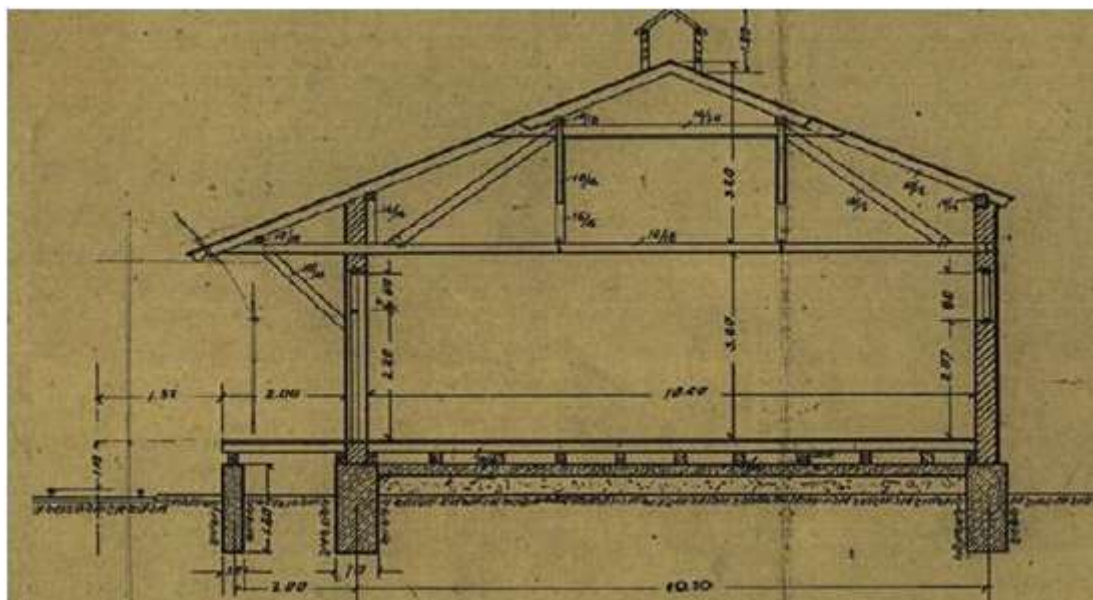
Rysunek nr 2: przekrój poprzeczny magazynu amunicyjnego nr 1.
