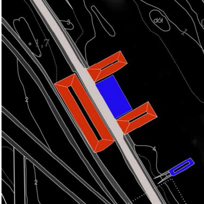
Rysunek nr 3: usytuowanie magazynu amunicyjnego 1 w terenie (kolor niebieski – magazyn amunicyjny oraz benzinmagazyn , kolor czerwony – wały ziemne).
