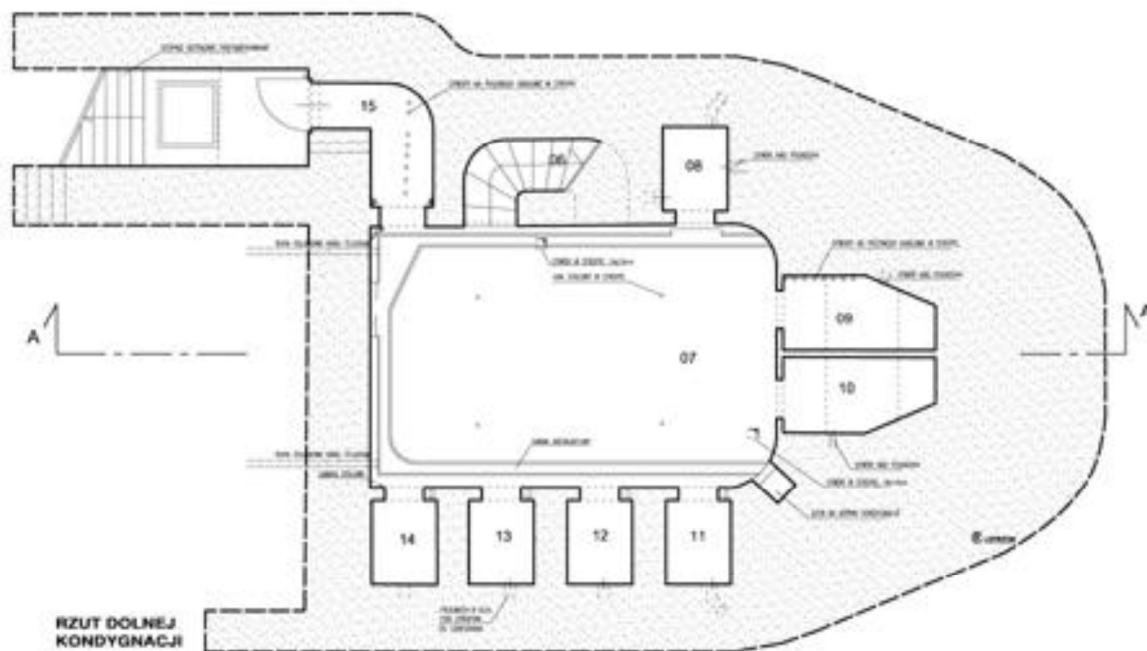
Rzut górnej i dolnej kondygnacji „Fortu” /źródło: Atelier Archifort Igor Strzokl
