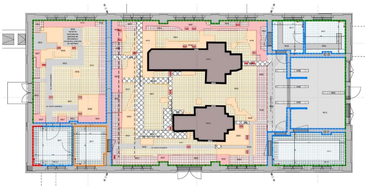
Ryc. 3. Projekt wykończenia posadzek i ścian budynku elektrowni na Westerplatte.
