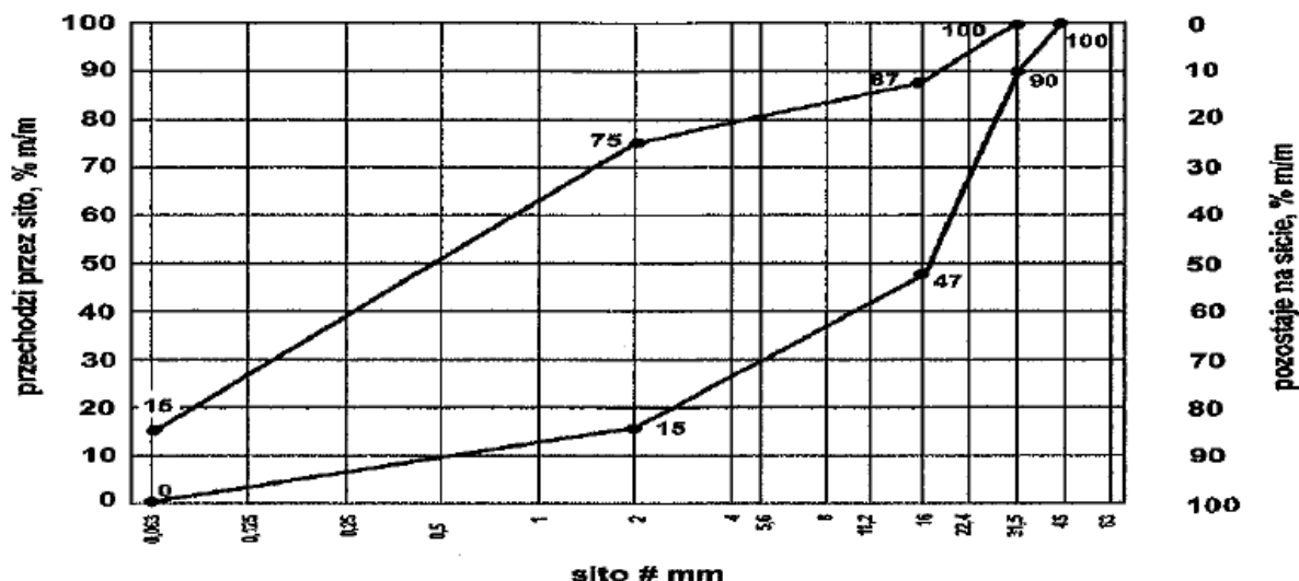
Rysunek 1. Mieszanka niezwiązana 0/31,5 do warstwy ulepszonego podłoża stabilizowanego georusztem 2.4. Parametry mieszanki niezwiązanej
