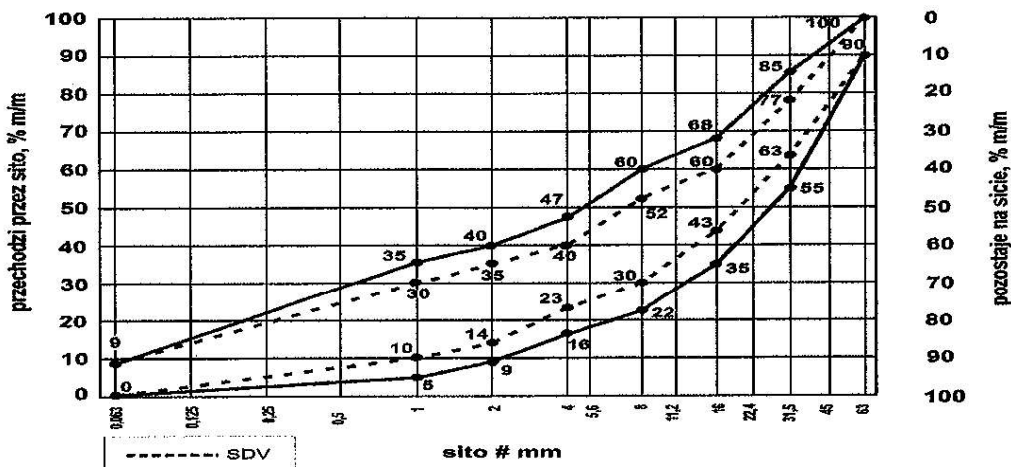
Rysunek 6. Mieszanka niezwiązana 0/63 do warstwy podbudowy zasadniczej
