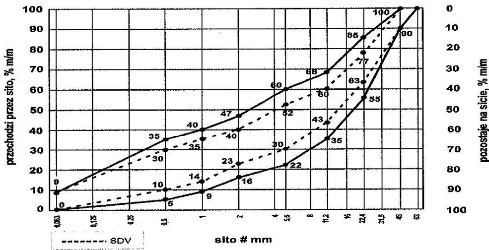
Rysunek 5. Mieszanka niezwiązana 0/45 do warstwy podbudowy zasadniczej
