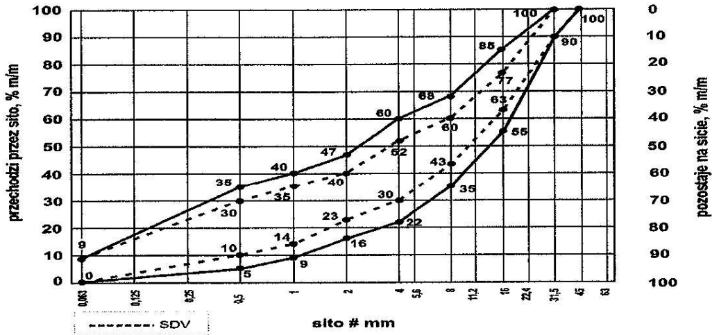
Rysunek 4. Mieszanka niezwiązana 0/31,5 do warstwy podbudowy zasadniczej
