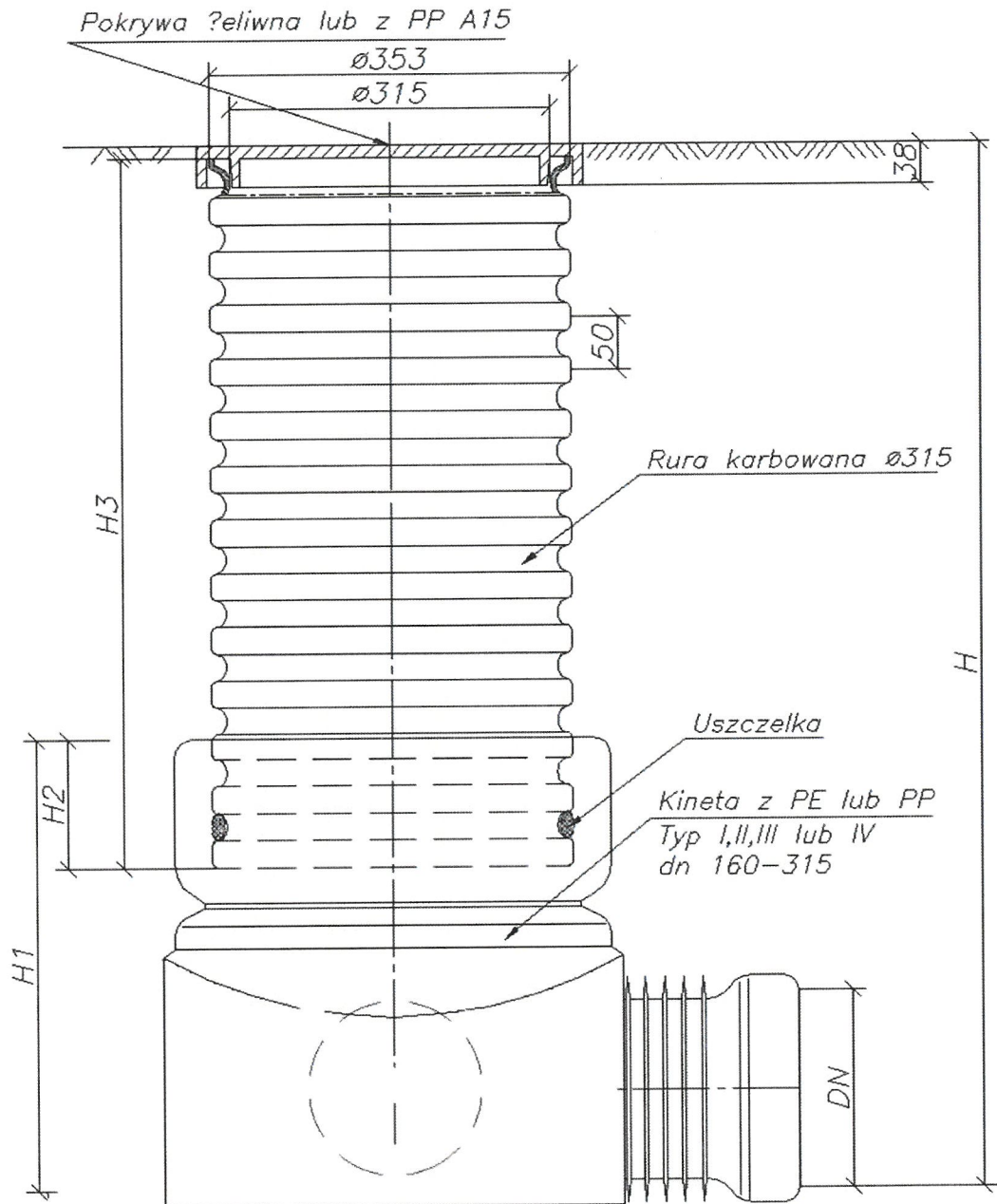
Studzienka inspekcyjna \varnothing 315 z pokrywą żeliwną lub z PP klasy A15
