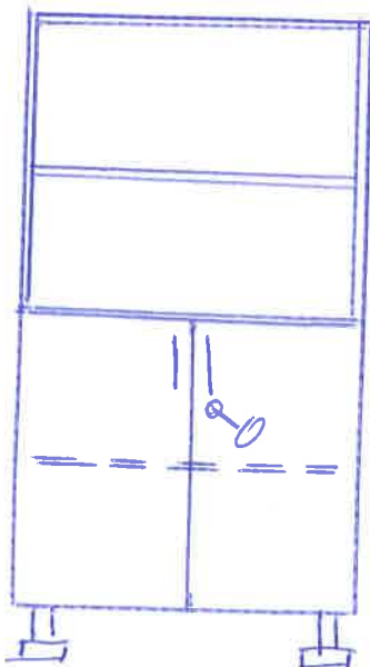
Szafa z półkami częściowo zamknięta na klucz 165 x 65 x 35
