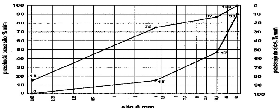
Rys. 7. Krzywe graniczne uziarnienia mieszanki kruszyw 0/63 mm do górnej warstwy podłoża ulepszanego
