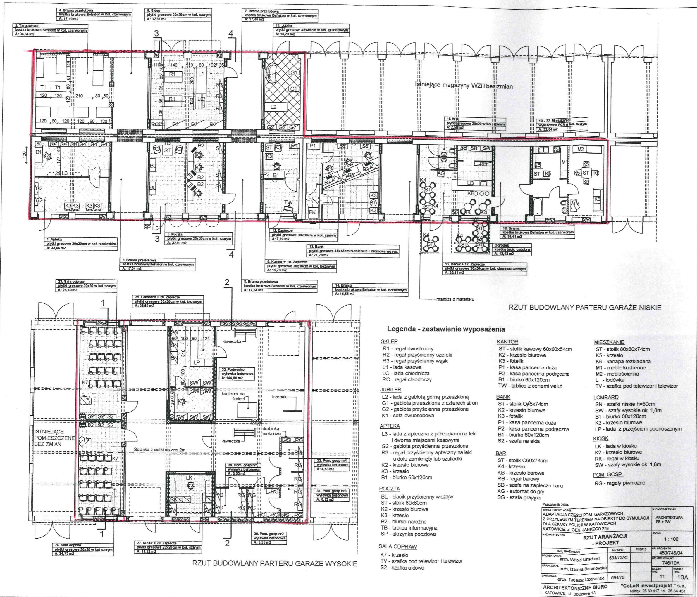
Rys. 3. Projekt aranżacji pomieszczeń WCS.
