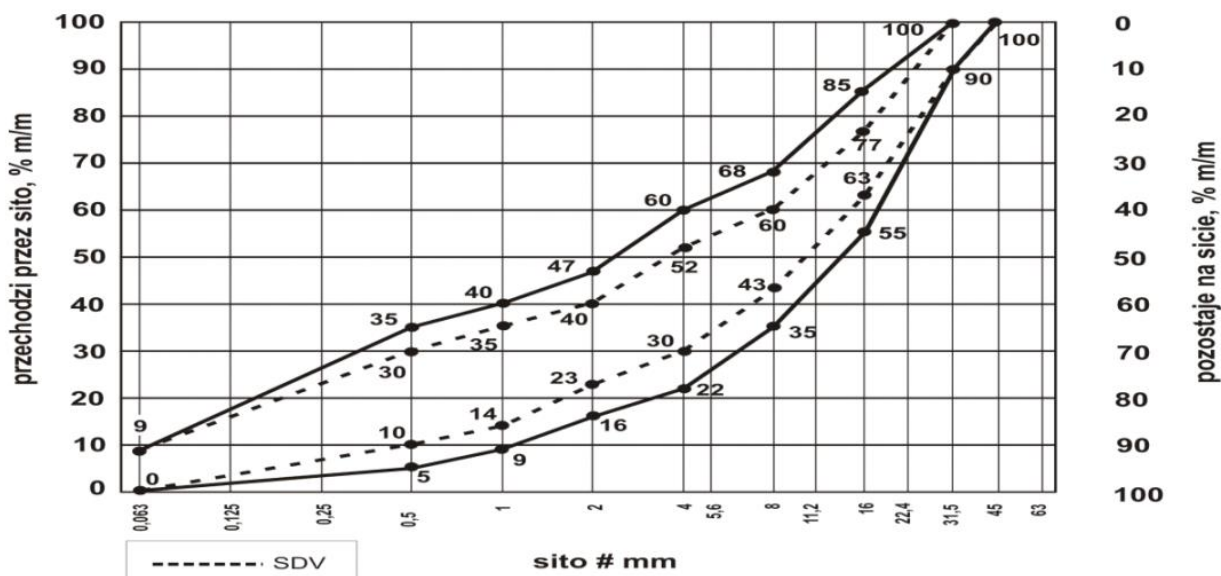
Rysunek 1. Uziarnienie mieszanki 0/31,5 do podbudowy zasadniczej
