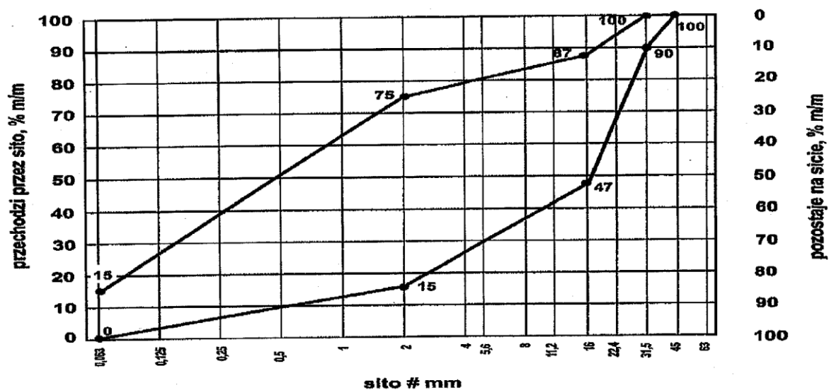
Rysunek 2. Uziarnienie mieszanki 0/31,5 na pobocza
