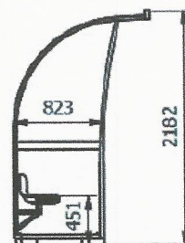
A-A ( 1 : 50 )
