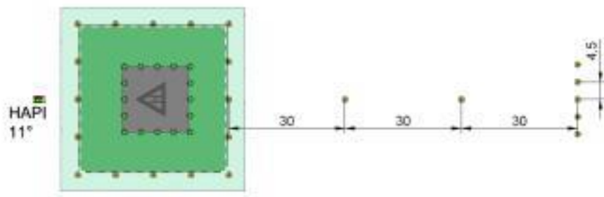
Rysunek 1. Schemat oświetlenia nawigacyjnego lotniska dla śmigłowców.
