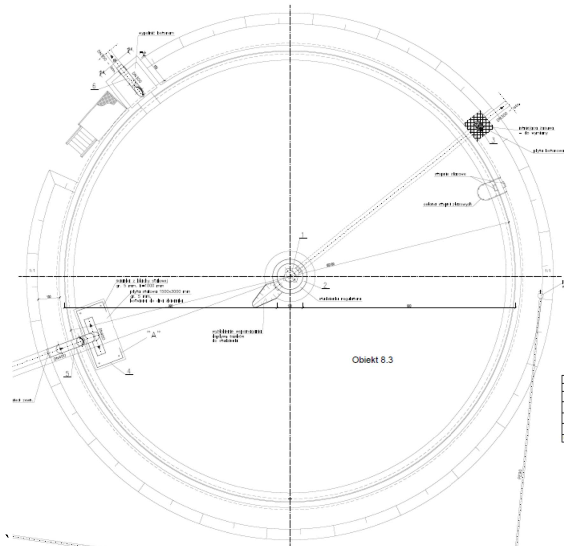
Rys. 2: Rzut zbiornika ob. 8.3
