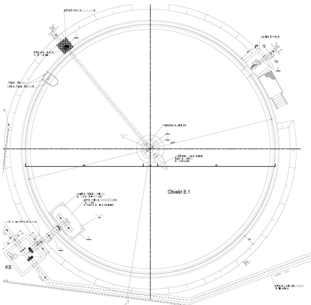
Rys. 1: Rzut zbiornika ob. 8.1
