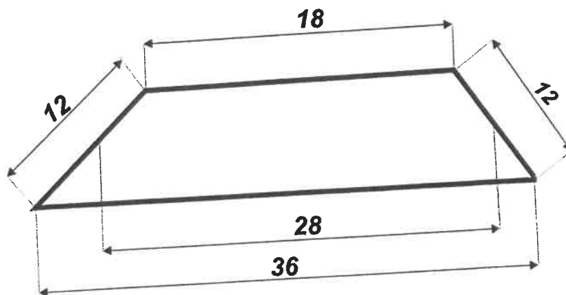
Rysunek 2 – Tkanina zasadnicza część II (środkowa)
