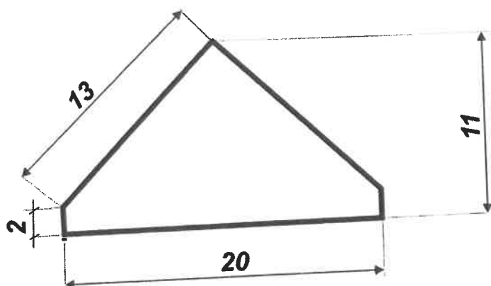
Rysunek 4 – Tkanina zasadnicza element odszycia dużego czuba
