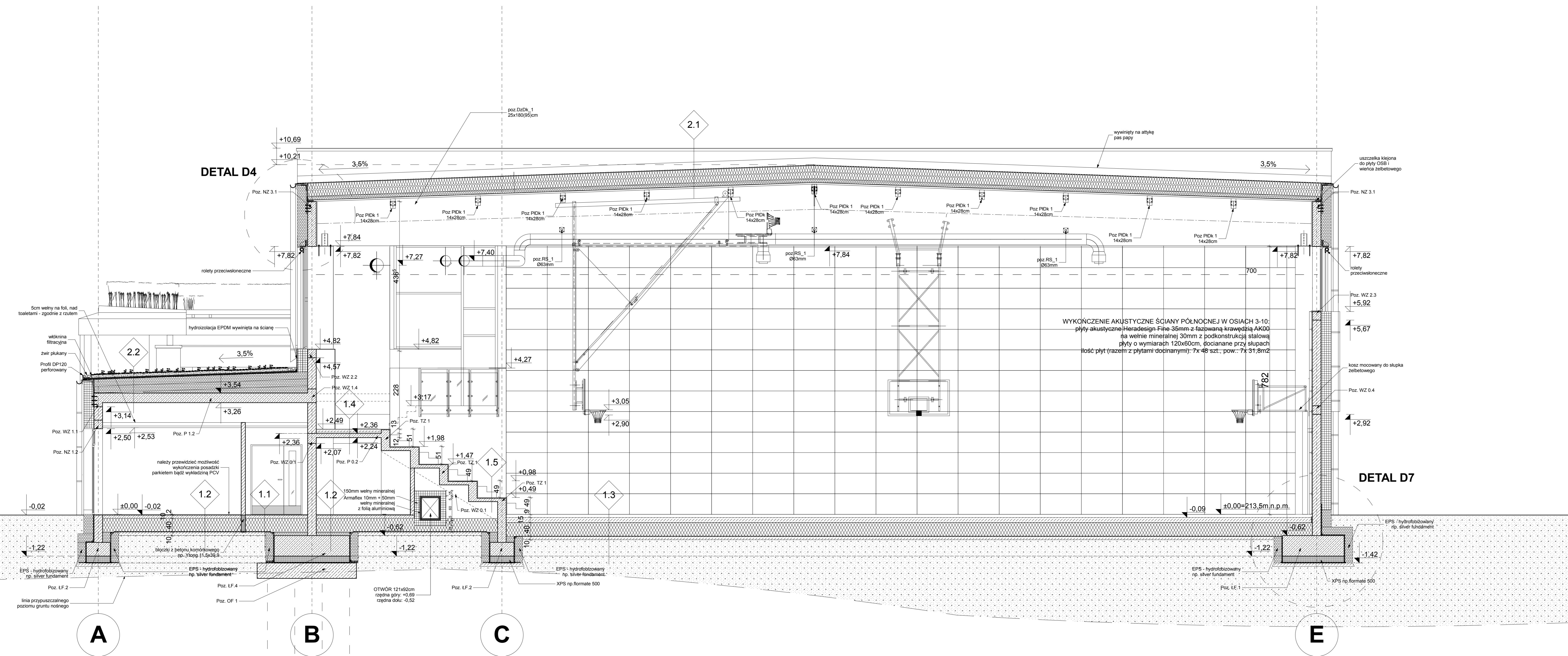
PRZEKRÓJ A-A
