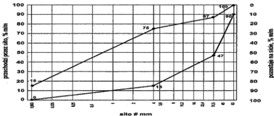
Rys.2 Mieszanka niezwiązana 0/63 do warstwy umocnionego pobocza z mieszanki niezwiązanej
