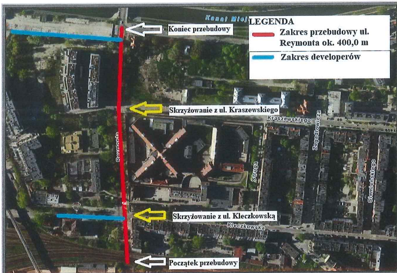
Rys. 2 Plan orientacyjny
