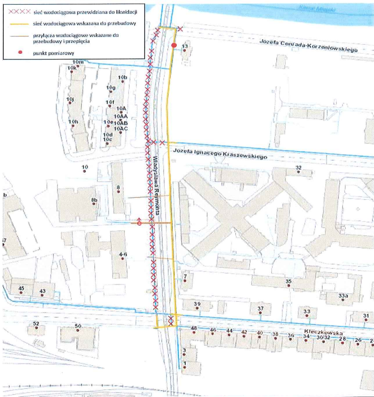
Rys. 3 Zakres budowy i przebudowy sieci wodociągowej w ul. W. Reymonta
