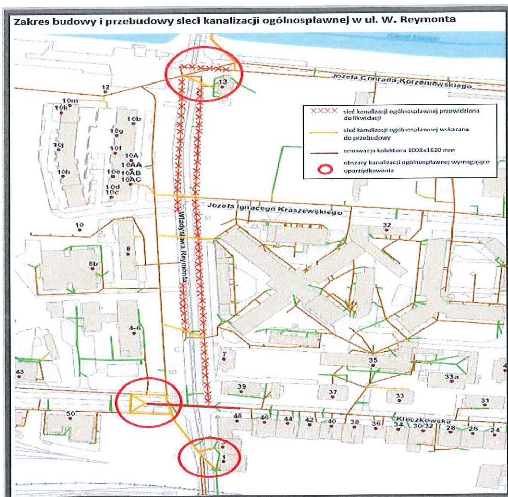
Rys. 4 Zakres budowy i przebudowy sieci kanalizacji ogólnospławnej w ul. W. Reymonta
