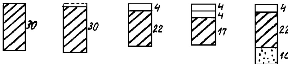
Rys. 4. Przyk6adowe wybrane konstrukcje nawierzchni utwardzonego pobocza z kruszywa łamanego niezwi6zanego
