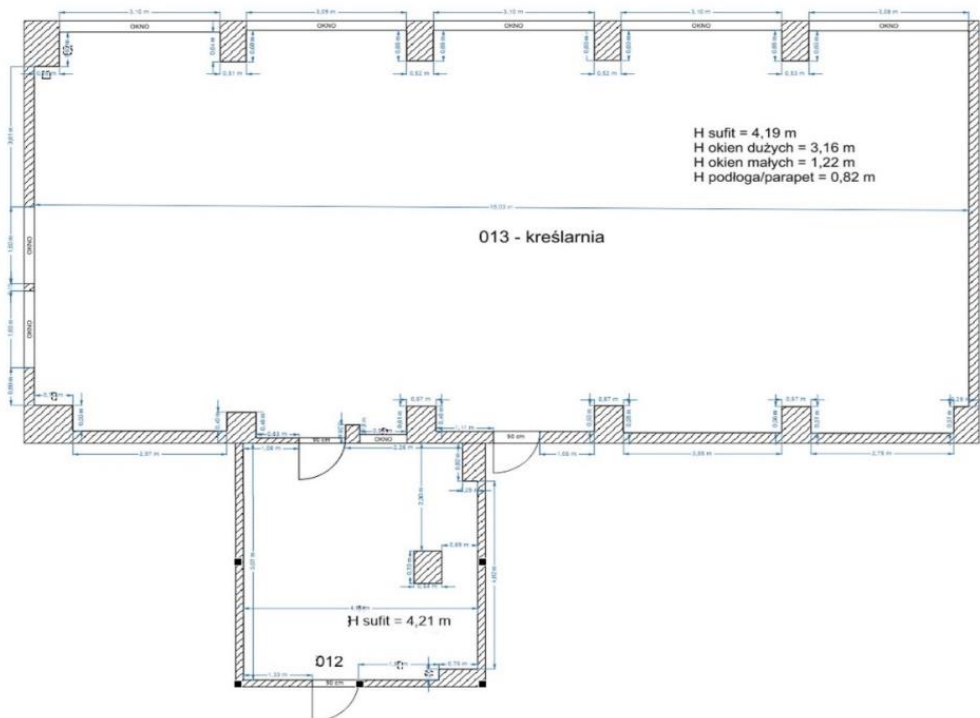
Rysunek 24 Rzut poglądowy z przybliżonymi wymiarami sali 012 i 013
